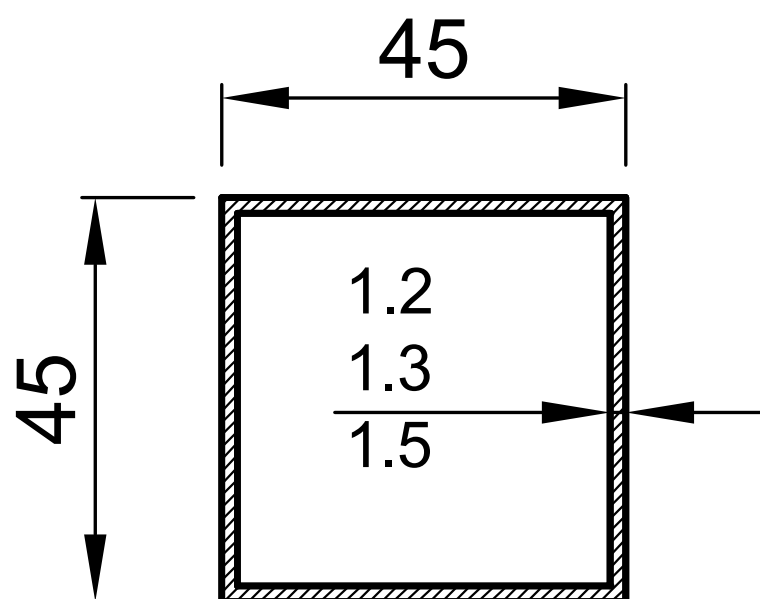
TQ45x45 AL CIJEV
