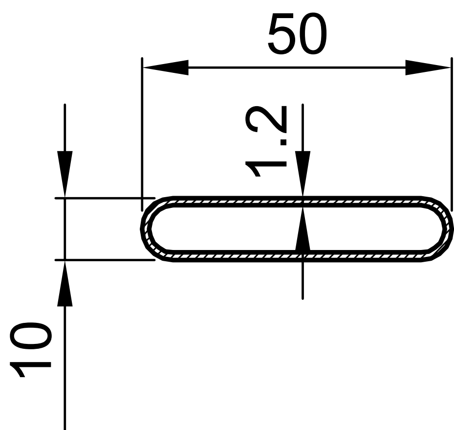
PM12593 ELIPSA 50x10x1.2 Težina: 0.292 kg/m
